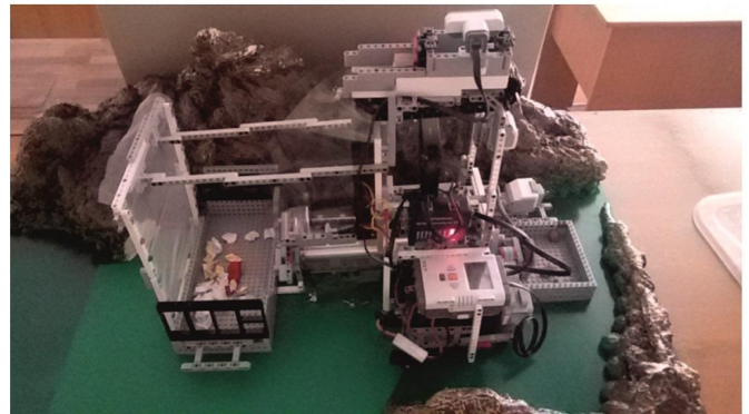
Сепаратор
