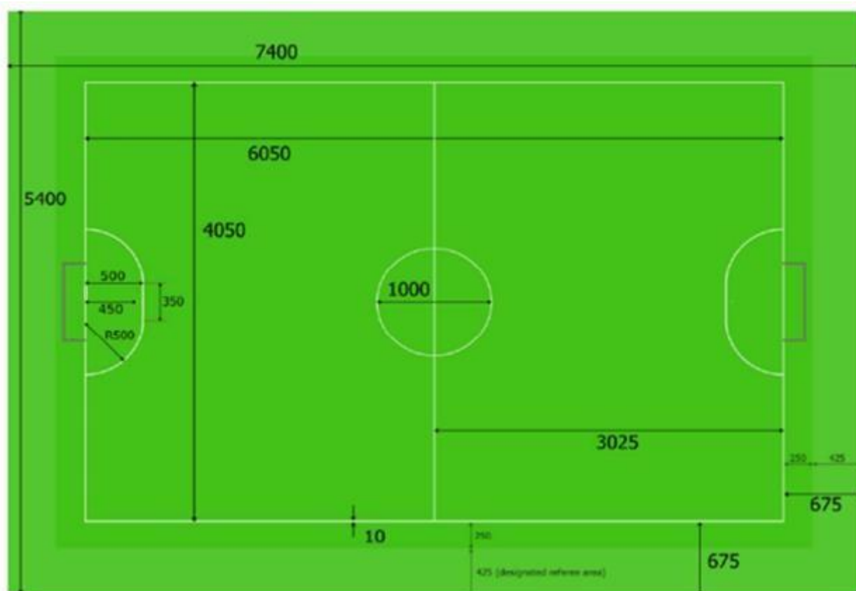
Рисунок 1. Схема поля
