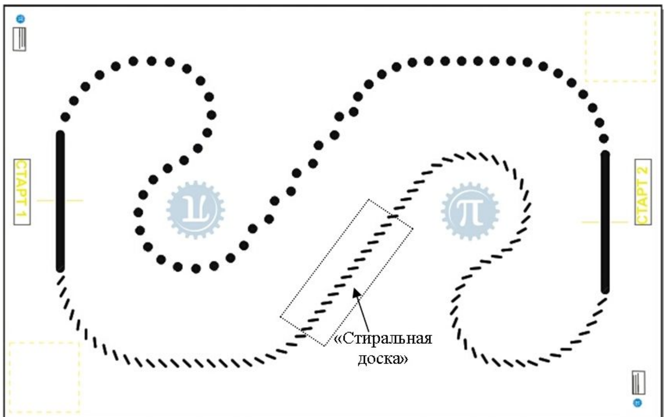
Рисунок 1. Расположение препятствия «стиральная доска».
