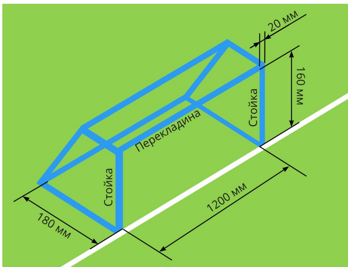
Рис. 3. Схема ворот
