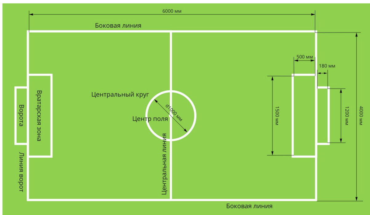
Рис. 2. Схема поля
