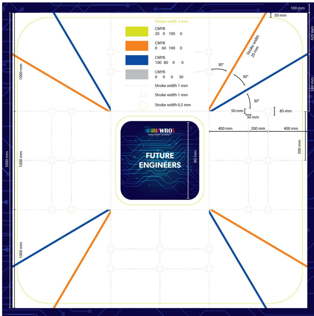
Рисунок 16. Карта игрового поля с размерами
